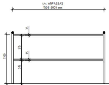
RÄCKE HÖGT - HÖJD 1100 MM TYPELEVATION RÄCKES-SEKTION Skala 1:20/A1, 1:40/A3
