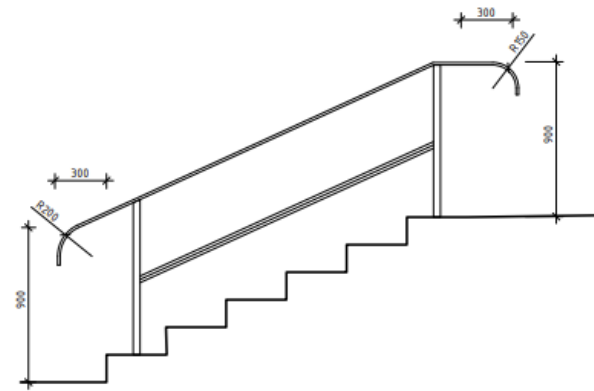
HANDEDARE - HÖJD 900 MM TYPELEVATION TRAPPA Skala 1:20/A1, 1:40/A3
