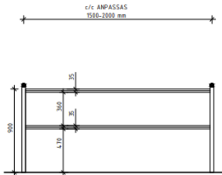
RÄCKE STANDARD - HÖJD 900 MM TYPELEVATION RÄCKES-SEKTION Skala 1:20/A1, 1:40/A3
