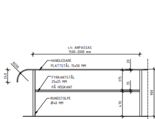
RÄCKE MED HANDEDARE - HÖJD 900 MM TYPELEVATION Skala 1:20/A1, 1:40/A3
