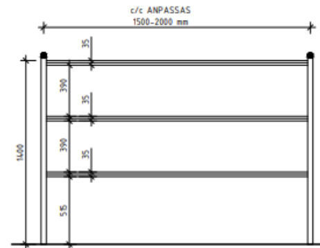
RÄCKE TRAFIK - HÖJD 1400 MM TYPELEVATION RÄCKES-SEKTION Skala 1:20/A1, 1:40/A3
