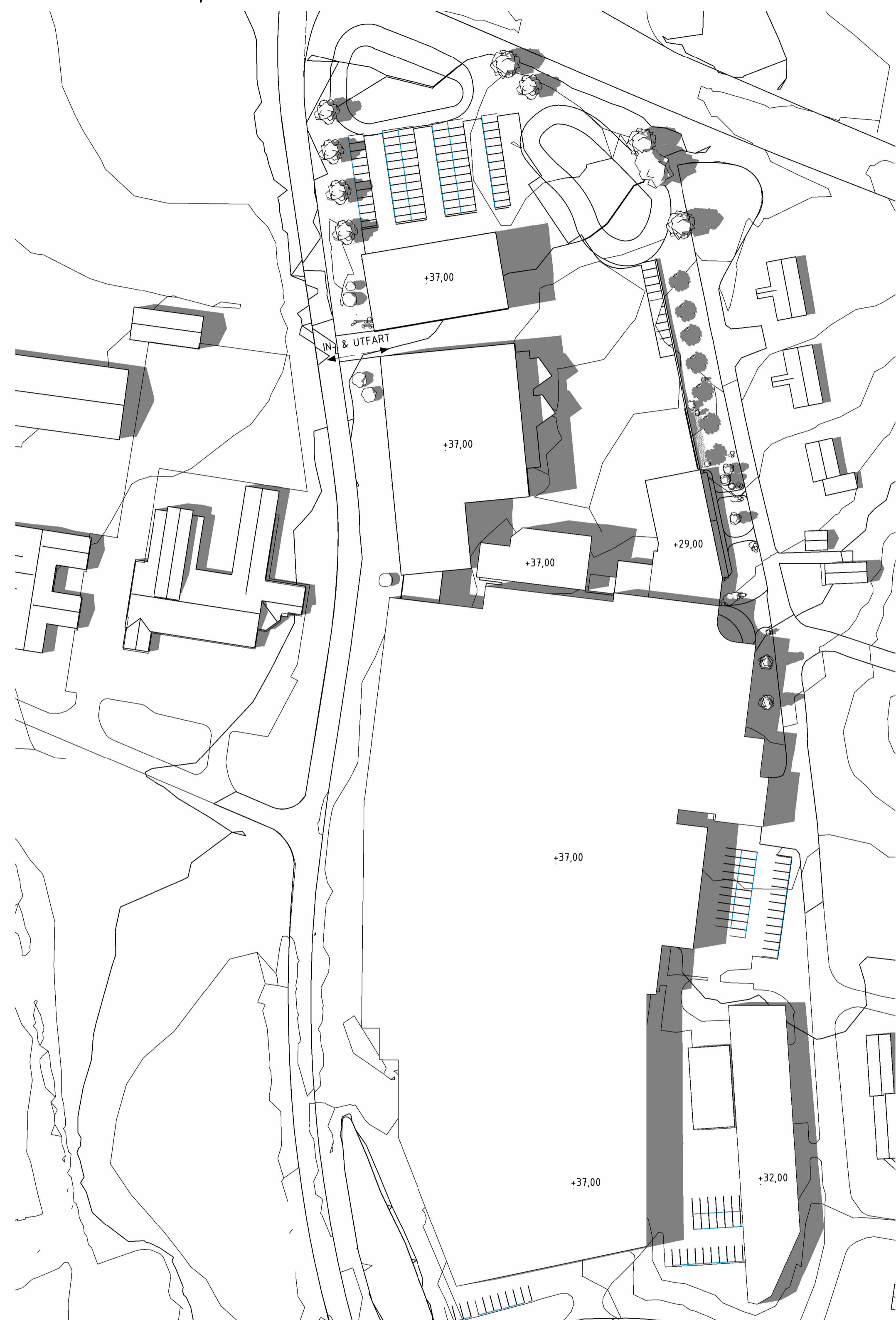
SOMMARSOLSTÅND, KL 15
