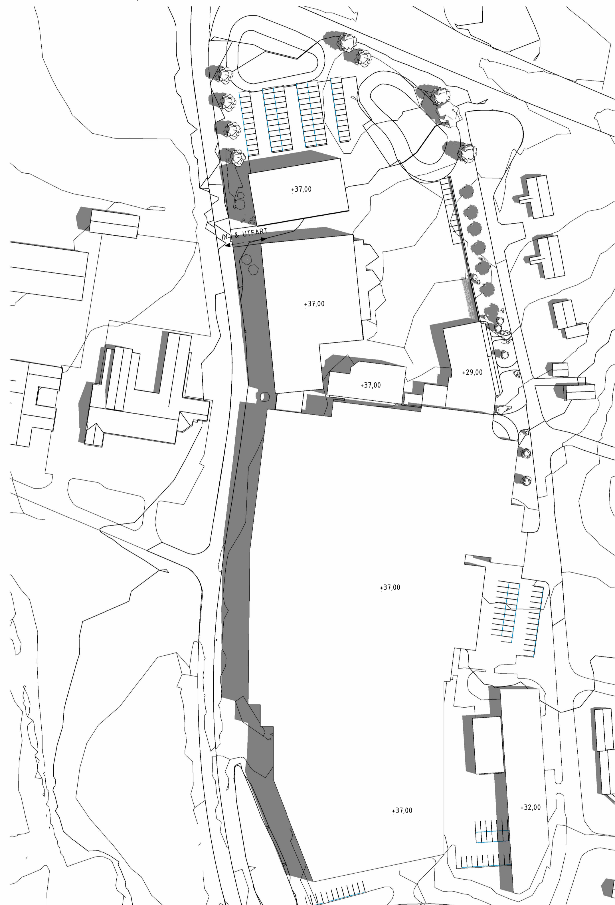
SOMMARSOLSTÅND, KL 9
