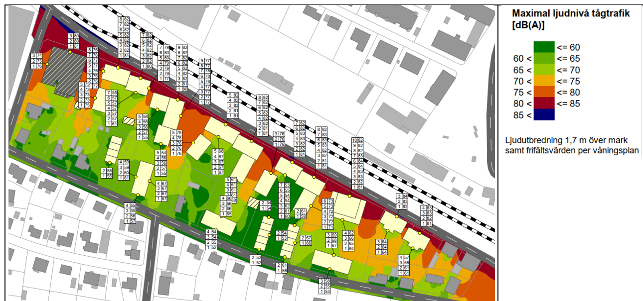
Figur 10. Detaljplaneområdet. Maximal ljudnivå från tågbuller med fördubblad tågtrafik jämfört med nuläget
