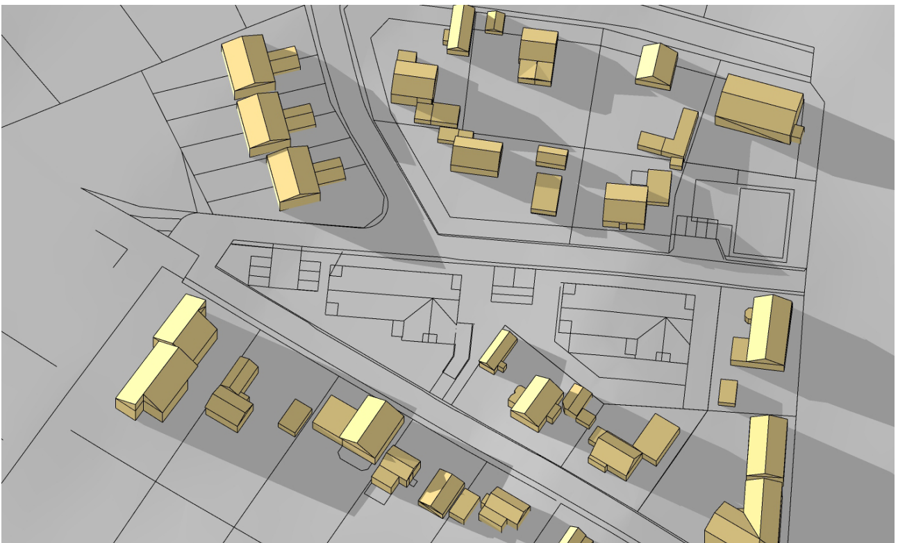
Vårdagjämning kl 17:00 - befintlig bebyggelse
