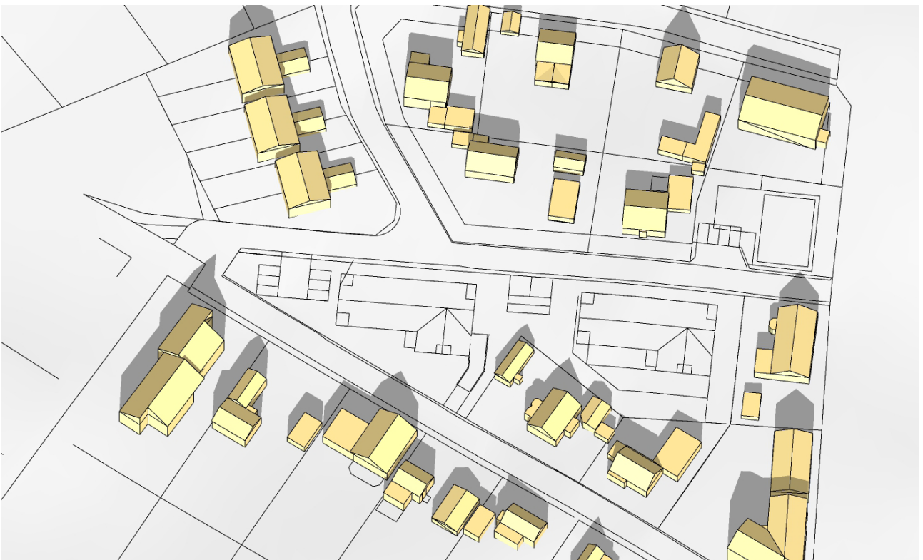
Vårdagjämning kl 10:00 - befintlig bebyggelse
