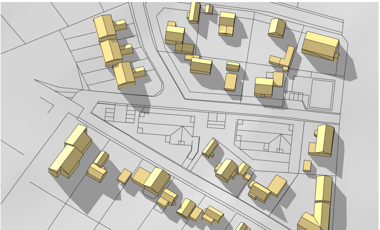
Sommarsolstånd kl 19:00 - befintlig bebyggelse
