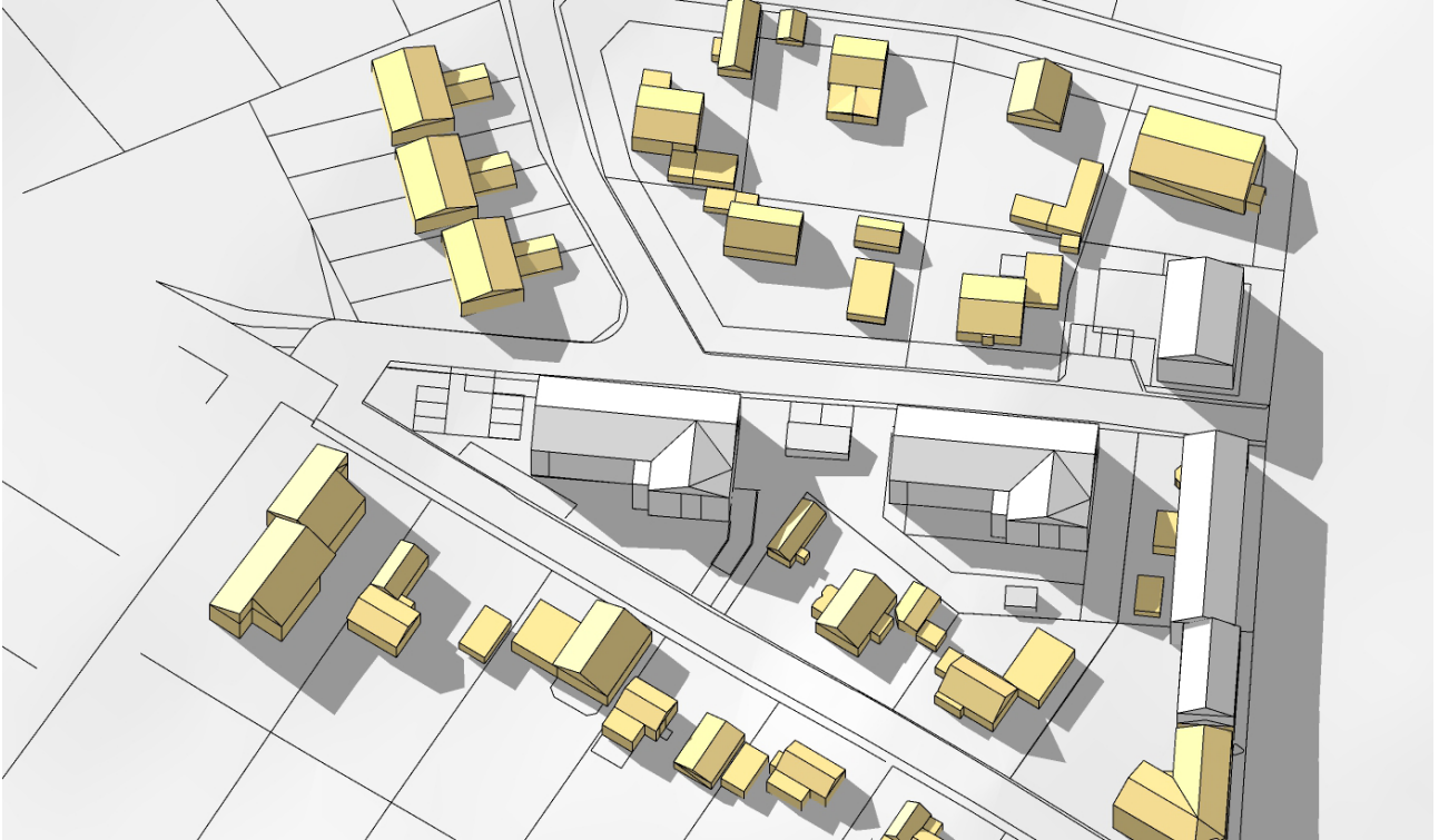
Sommarsolstånd kl 18:00 - föreslagen bebyggelse
