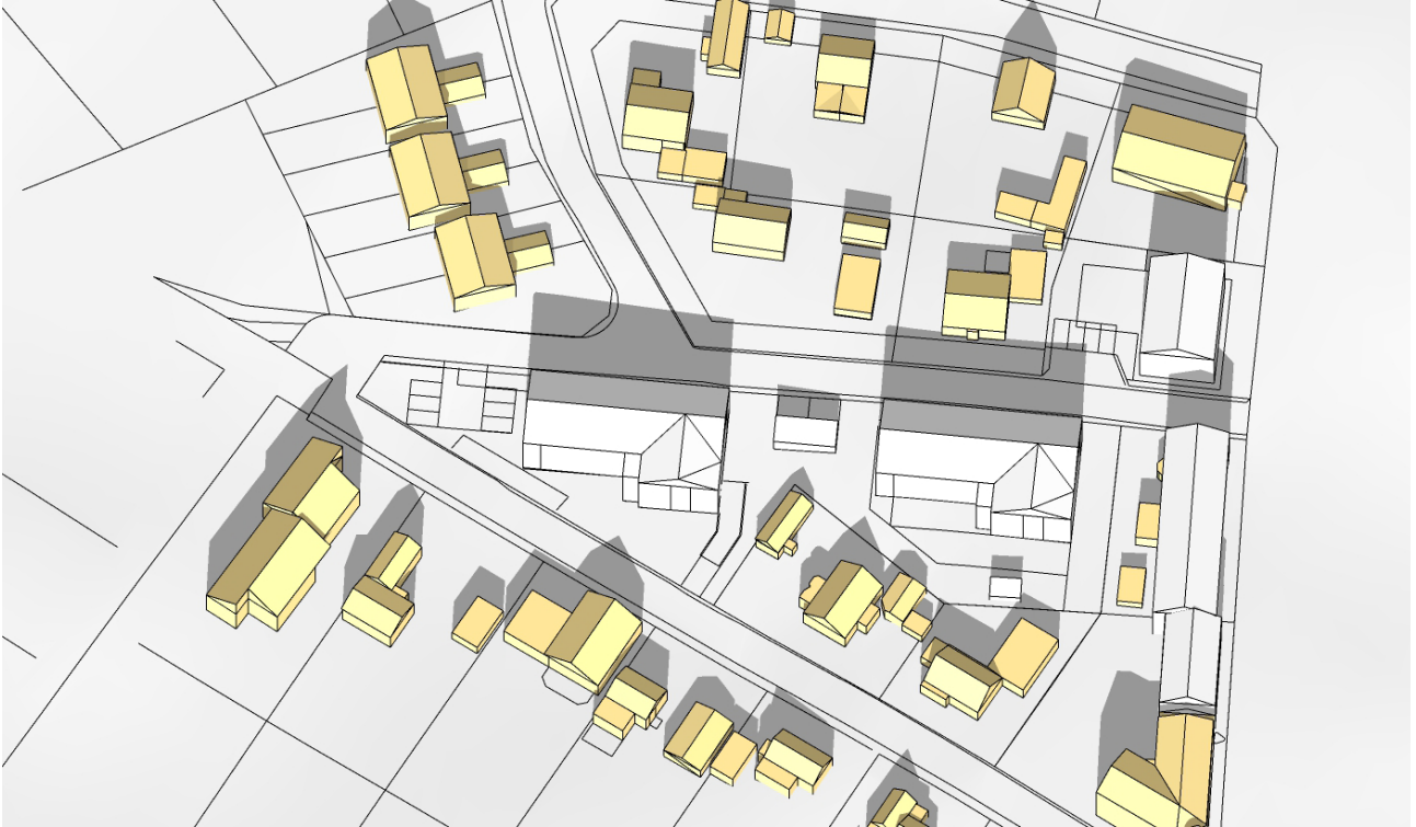
Vårdagjämning kl 10:00 - föreslagen bebyggelse
