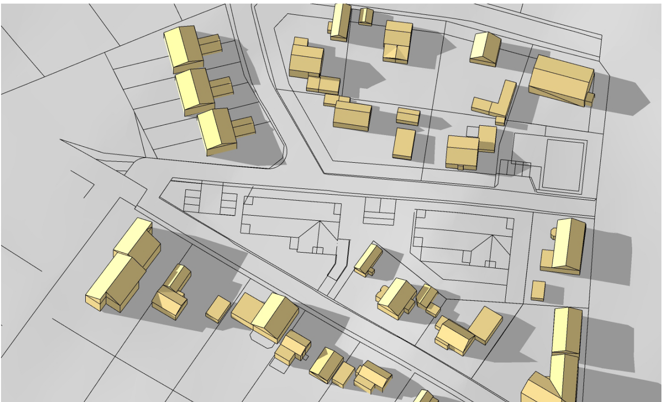
Vårdagjämning kl 16:00 - befintlig bebyggelse
