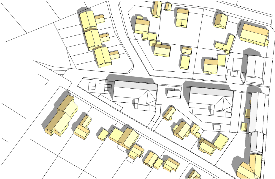
Sommarsolstånd kl 10:00 - föreslagen bebyggelse
